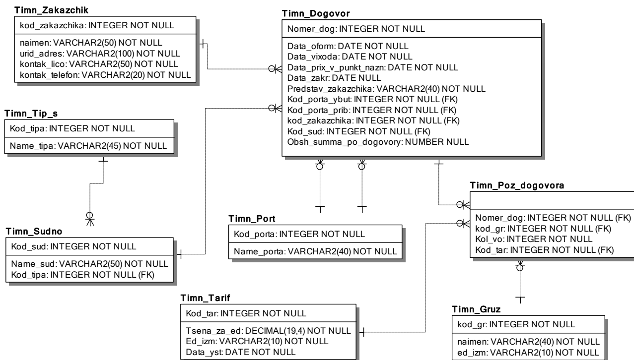
Рисунок 2.2 - Физическая модель данных
